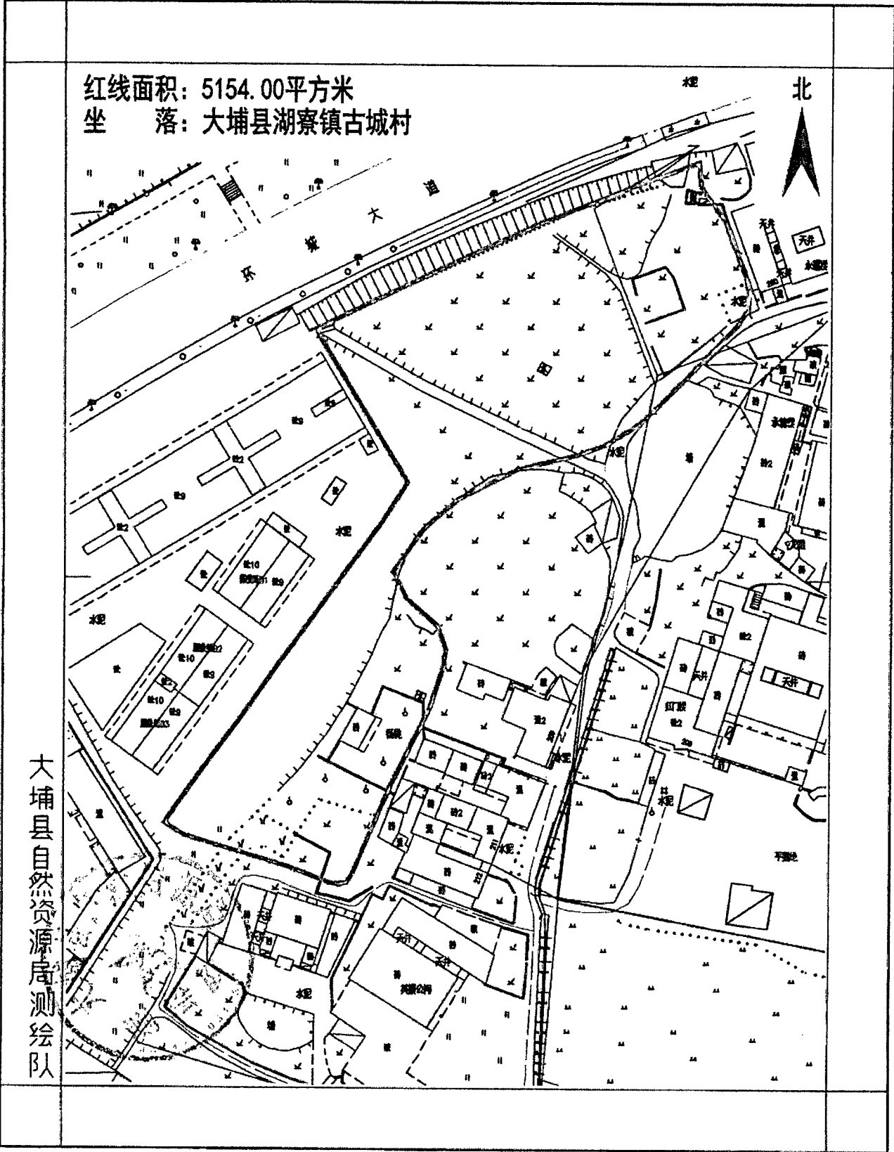
大埔县2021年度第一批次城镇建设用地图(古城村)勘测定界图
