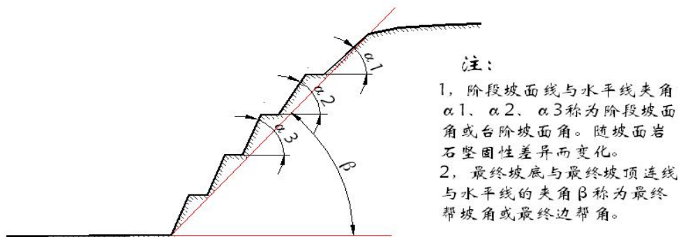
露天采矿场(坑)阶段坡面角与最终帮坡角
