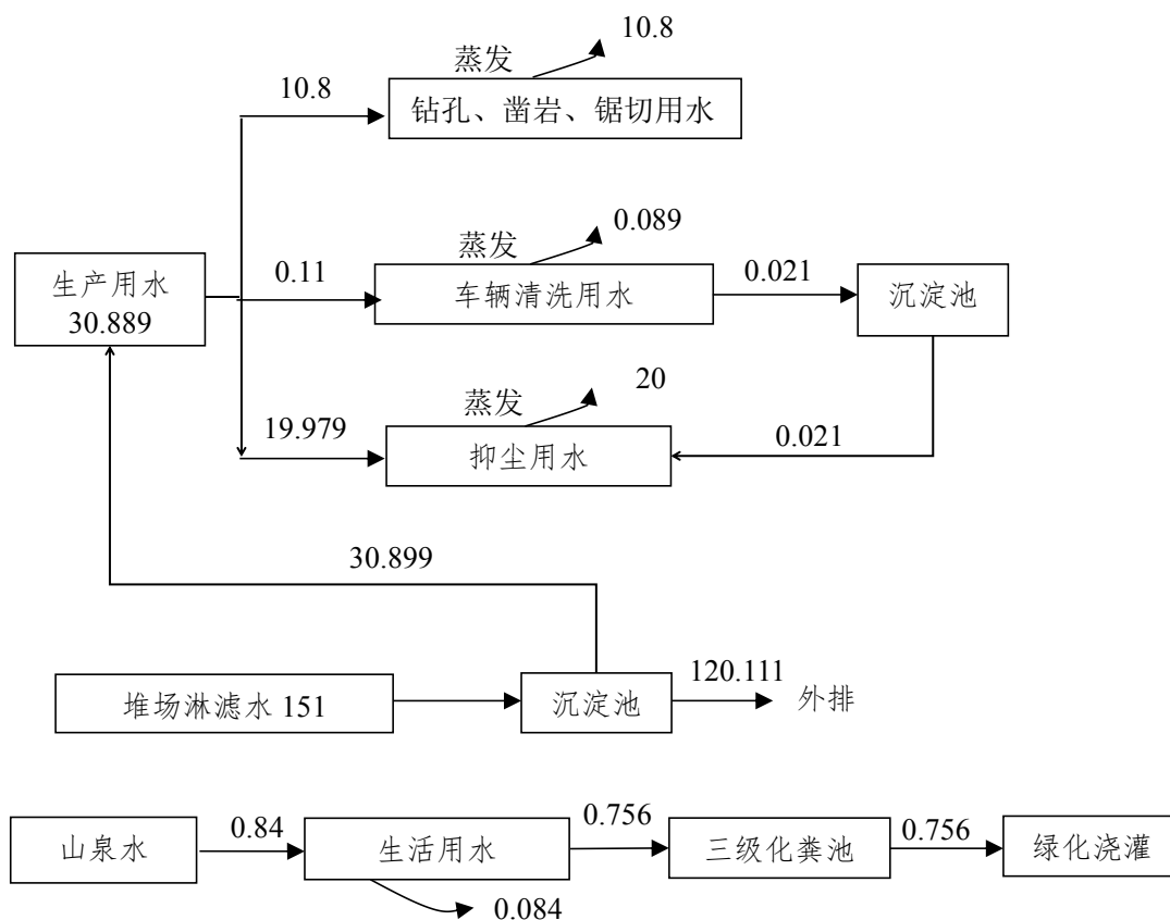
图 4-2 改建后雨季期水平衡图 (m 3 /d)
