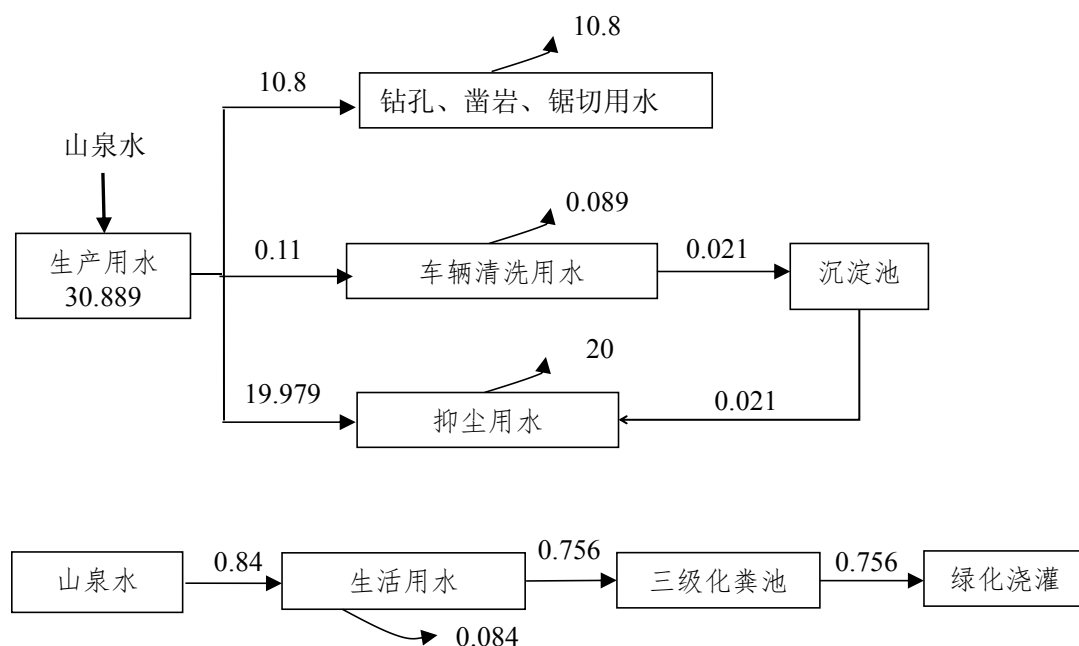
图 4-3 改建后非雨季期水平衡图 (m³/d)
