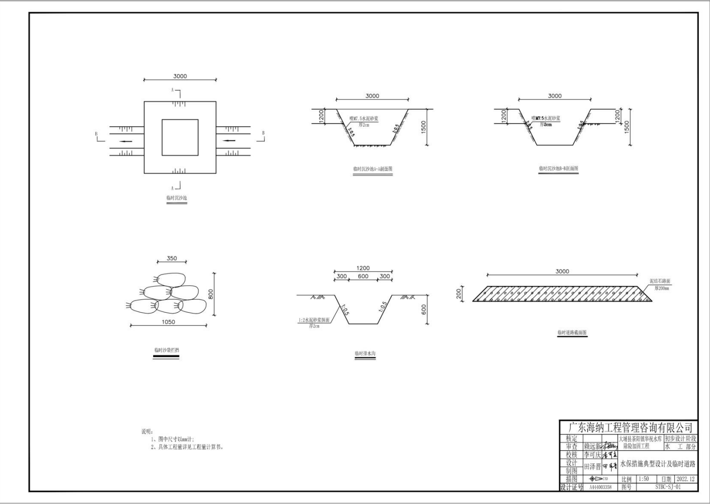
附图 16 生态环境典型措施设计图
