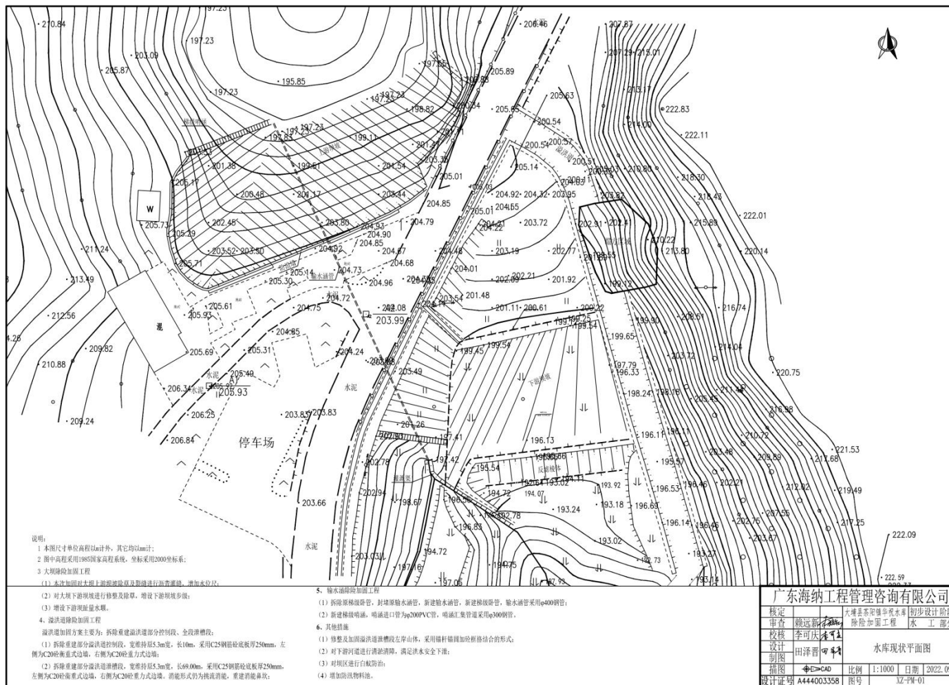
附图 12 水库现状平面图
