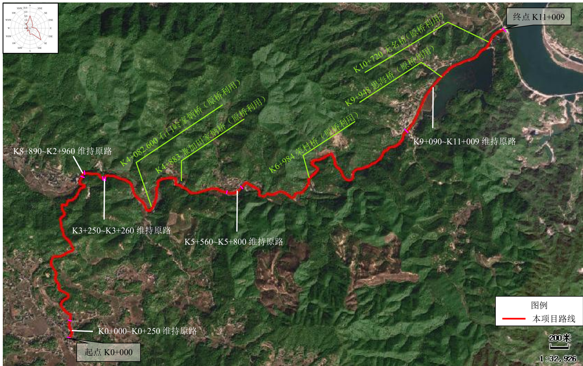
附图 2 项目总平面图
