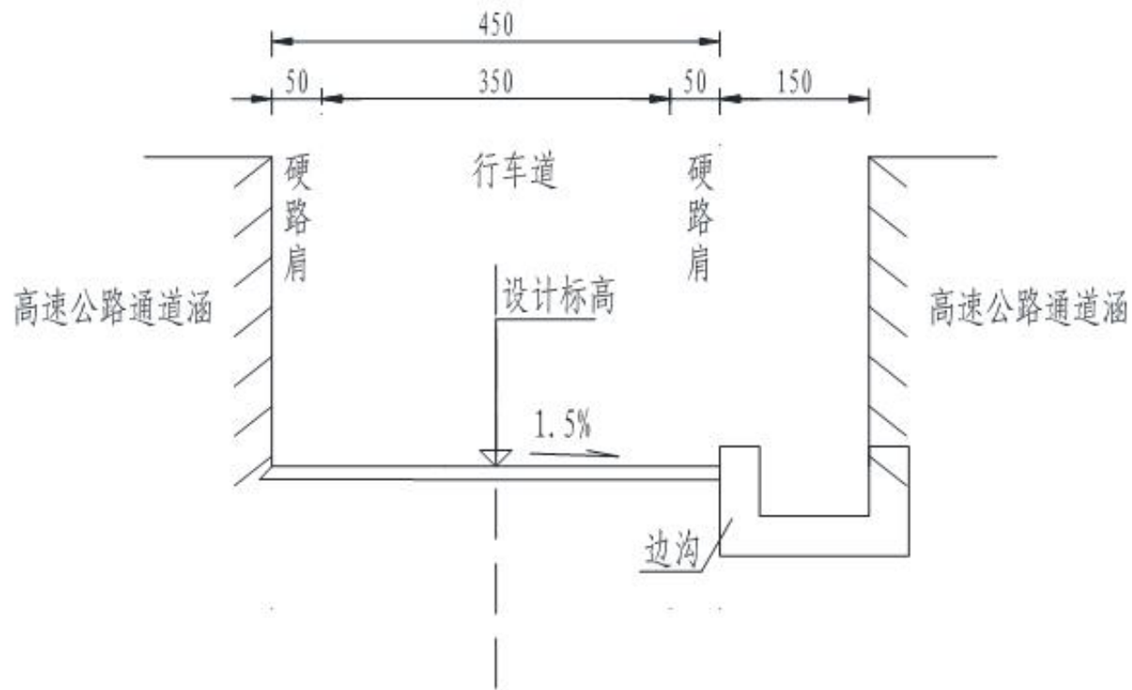
附图 5-1 路基标准断面设计图 (4.5m 路基标准断横面-K2+890~K2+960、K3+250~K3+260、K5+560~K5+800 用地受限段)
