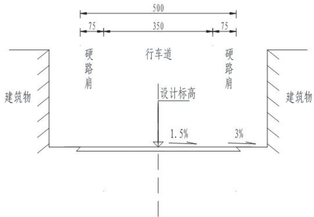
附图 5-2 路基标准断面设计图 (5m 路基标准断横面-K0+000~K0+250 用地受限段)
