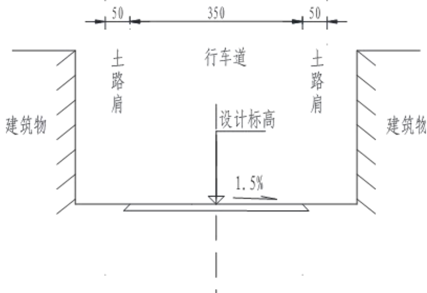
图 2-2 路基标准横断面示意图（路基宽度 4.5m）
